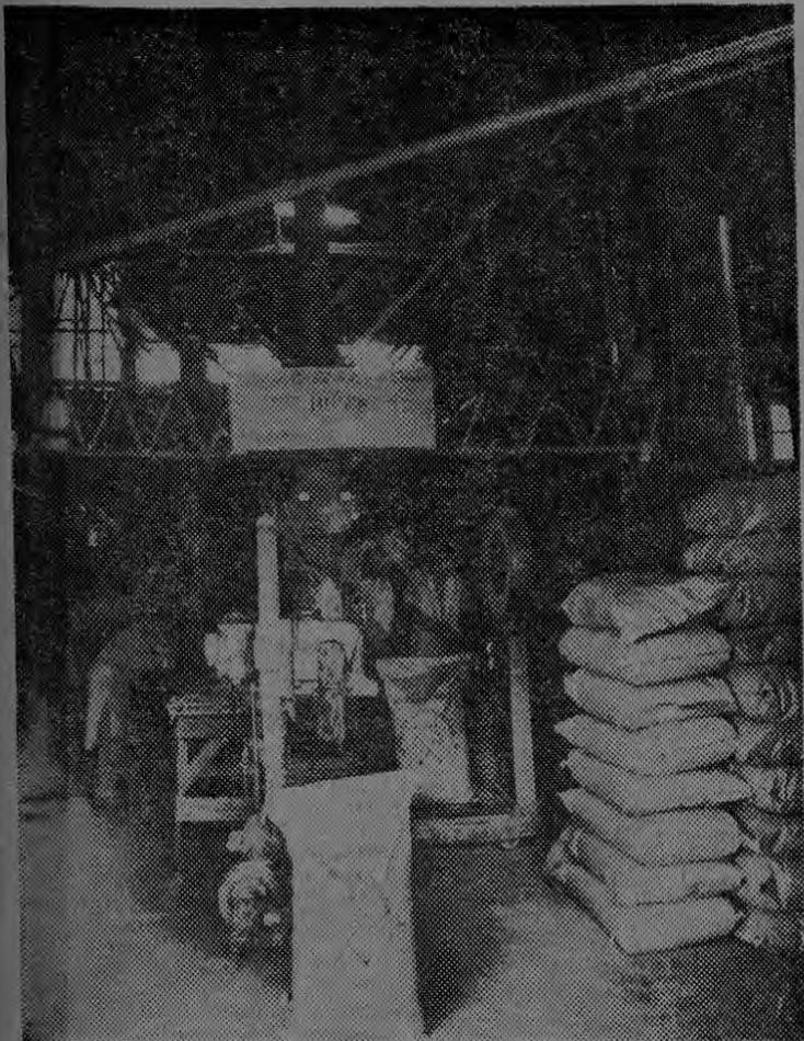
Una sección de la maquinaria confeccionadora de alimentos en PELLETS, con sus respectivas TOLVAS y ELEVADORES DE HUACAL.
